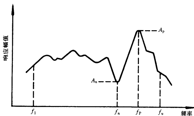
图 1 峰谷幅值比的确定
