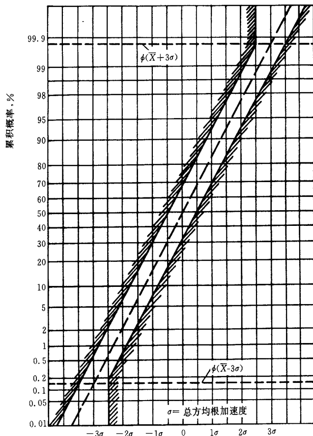
图3 瞬时加速度分布的容差带
