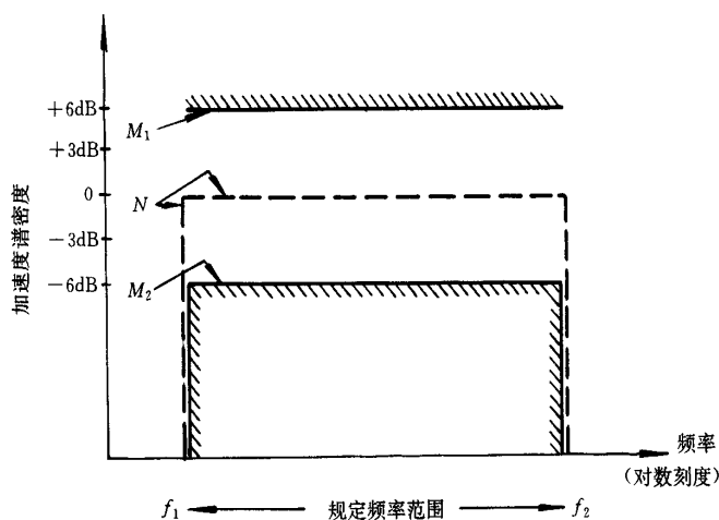
M_1 —容差上限,中再现性; M_2 —容差下限,中再现性; N —规定的加速度谱密度的标称值
