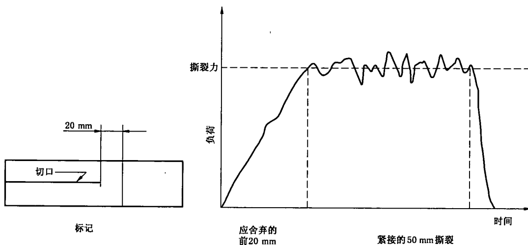
图4 曲线平稳部分的负荷-时间图
