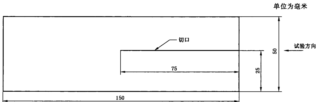
图 1 试样
